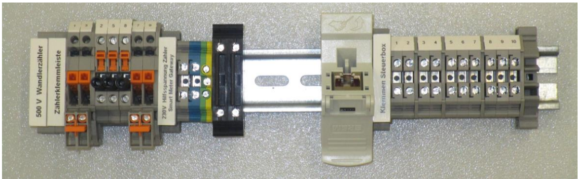
Abbildung 5: Zählerklemmleiste Wandlermessung 500 V
