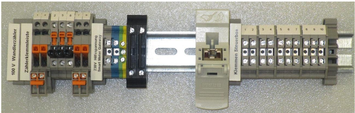
Abbildung 67: Zählerklemmleiste Mittel- und Hochspannung
