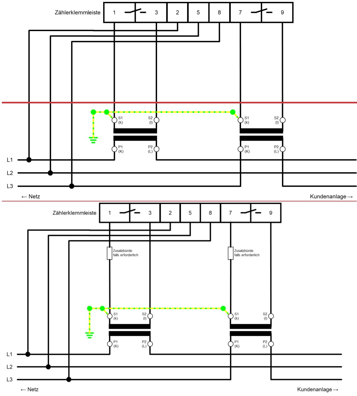
Abbildung 1143 1143: Verdrahtung 500 V Wandlermessung
