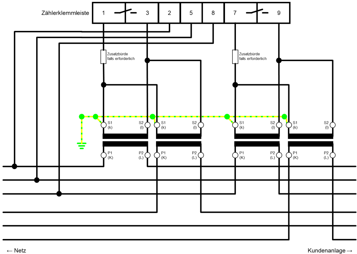
Abbildung 1042: Verdrahtung 500 V Wandlermessung für redundanten Netzanschluss NS/N
