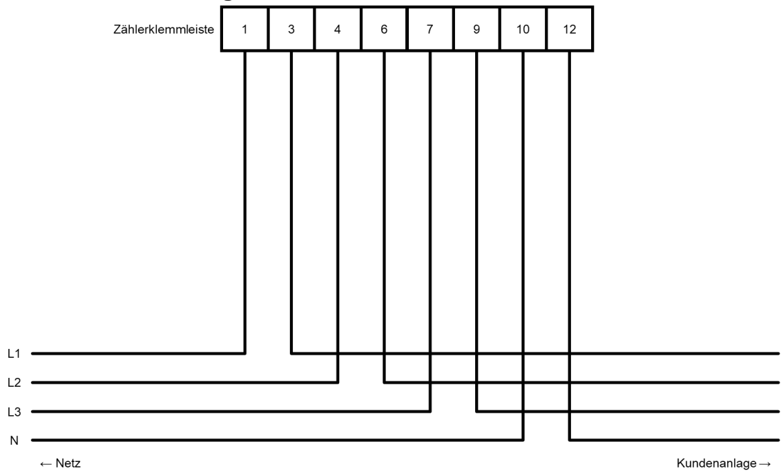
Abbildung 89: Verdrahtung 400 V direkte Messung
